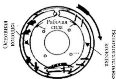
Рис 6-6 Торможение при движении назад
