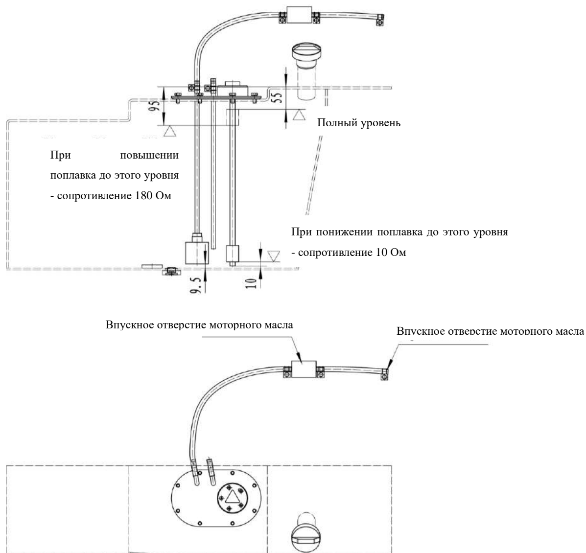
Рис 1-4 Топливный бак (Бензиновый вилочный погрузчик)
